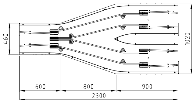
Boven aanzicht
